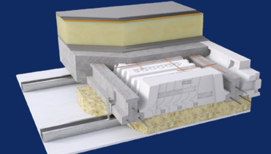
Plancher Terrawatt avec Isorupteurs dB
