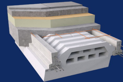
Plancher Duo Isoleader et chape flottante
