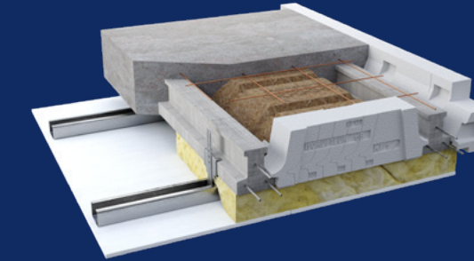
Plancher Silence avec Isorupteurs dB ou Isorupteurs dB EI30
